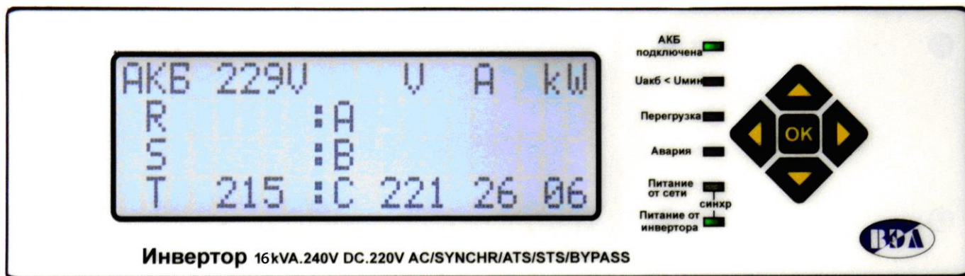
Рис. 2 Расположение органов управления и индикации инвертора
