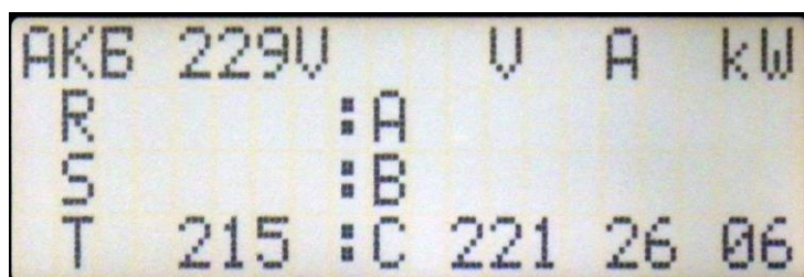
Рис. 5. Экран дисплея инвертора
