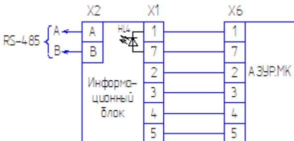
Рисунок 3 — Схема подключения информационного блока БИН.4МК к аппарату АЗУР.4МК
