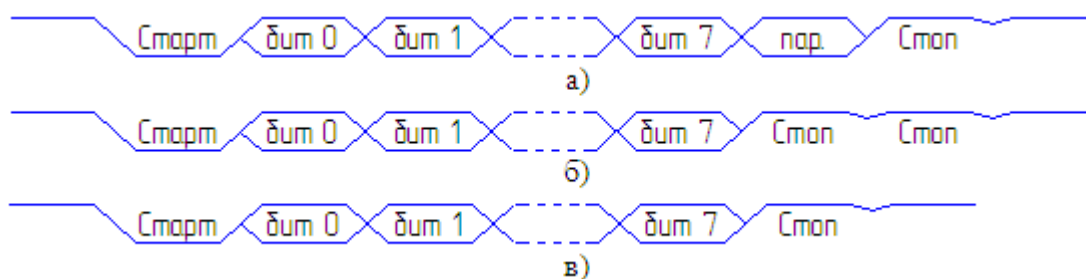
Рисунок 4 — Формат байта: а) с контролем паритета, б) без контроля паритета (1 стоп бит), в) без контроля паритета (2 стоп бита)
