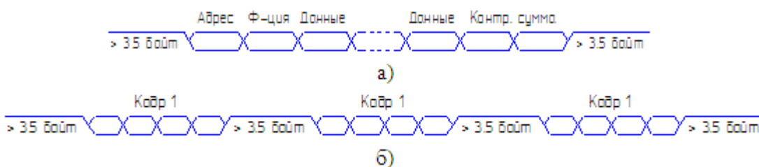
Рисунок 5 — Формат кадра: а) одного, б) трех последовательных кадров
