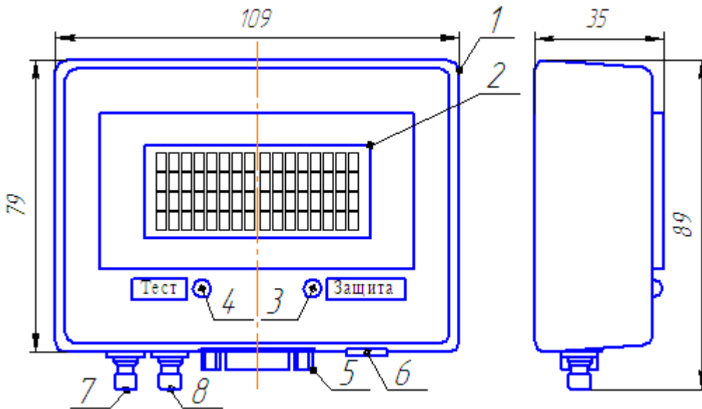
Рисунок 2 — Информационный блок БИН.4МК
