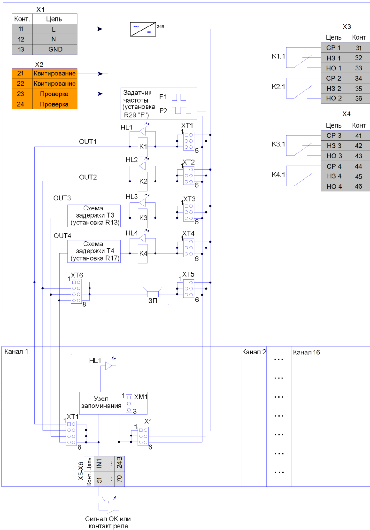
Рисунок 2.3 – Схема работы устройства УАС-16(УАС-16MI)
