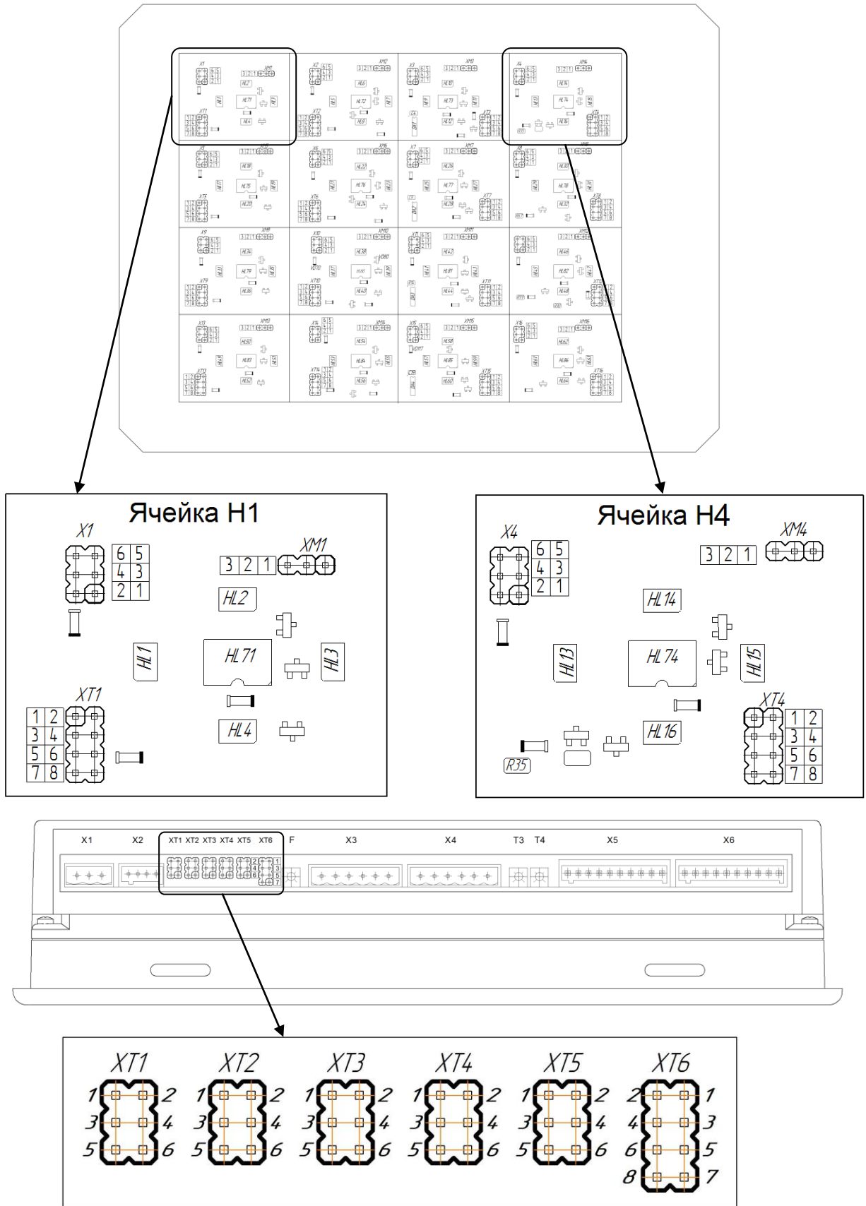
Рисунок 2.2 – Расположение перемычек на плате устройства УАС-16(УАС-16М)
