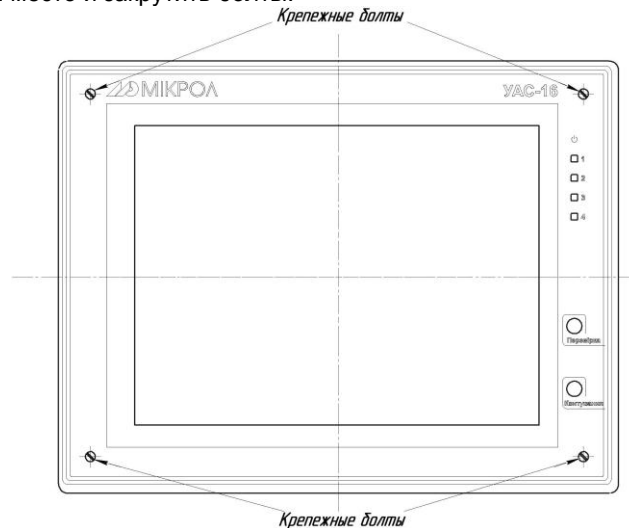
Рисунок 1.1 – Размещение крепежных болтов на передней панели УАС-16 (УАС-16MI)
