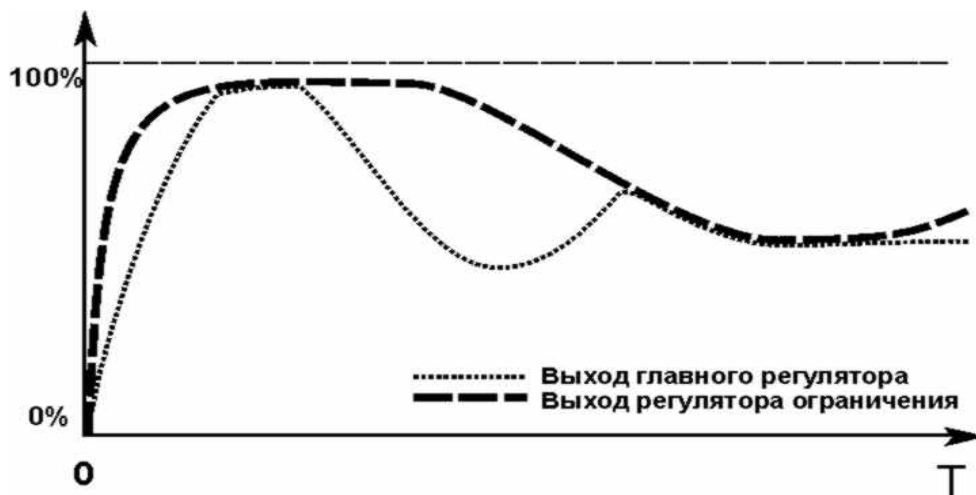
Рисунок 5.7 - График работы override регулятора в режиме ограничения по максимуму
