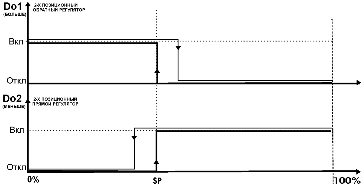
Рисунок В.9 - График работы 3-х позиционного регулятора с использованием гистерезиса но без зоны нечувствительности 2-х позиционного прямого и обратного регулятора.
