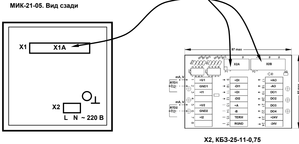
Рисунок Б.1 - Подключение клеммно-блочного соединителя КБ3-25-11-0,75 к регулятору МИК-21-
