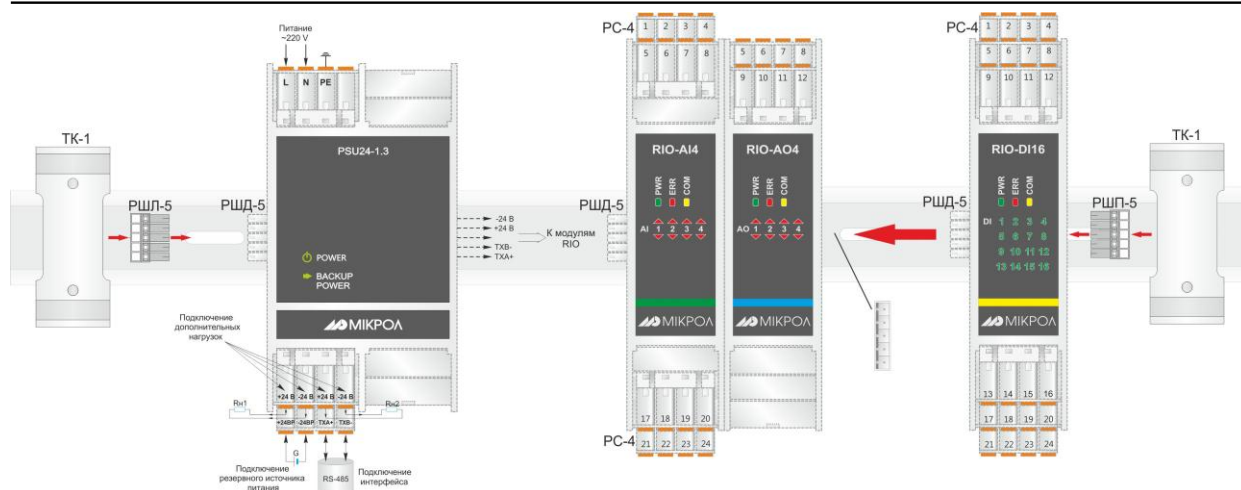
Рисунок Б.3 - Схема внешних соединений RIO-DI16 с блоком питания и другими модулями
