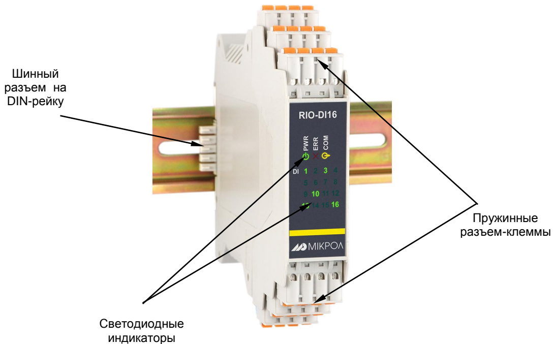
Рисунок. 3.1 - Внешний вид модуля дискретного ввода RIO-DI16
