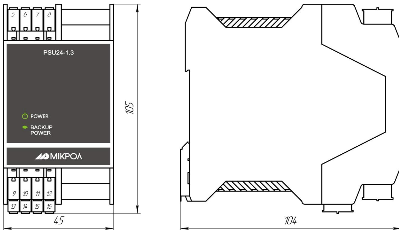
Рисунок 1.1 – Внешний вид и габаритные размеры PSU24-1.3
