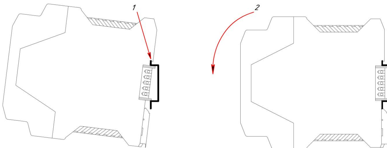
Рисунок 4.1 – Схема крепления блока питания на DIN-рельс
