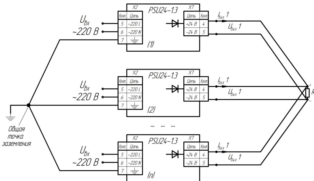
Рисунок 2.1 - Параллельное соединение блоков питания PSU24-1.3
