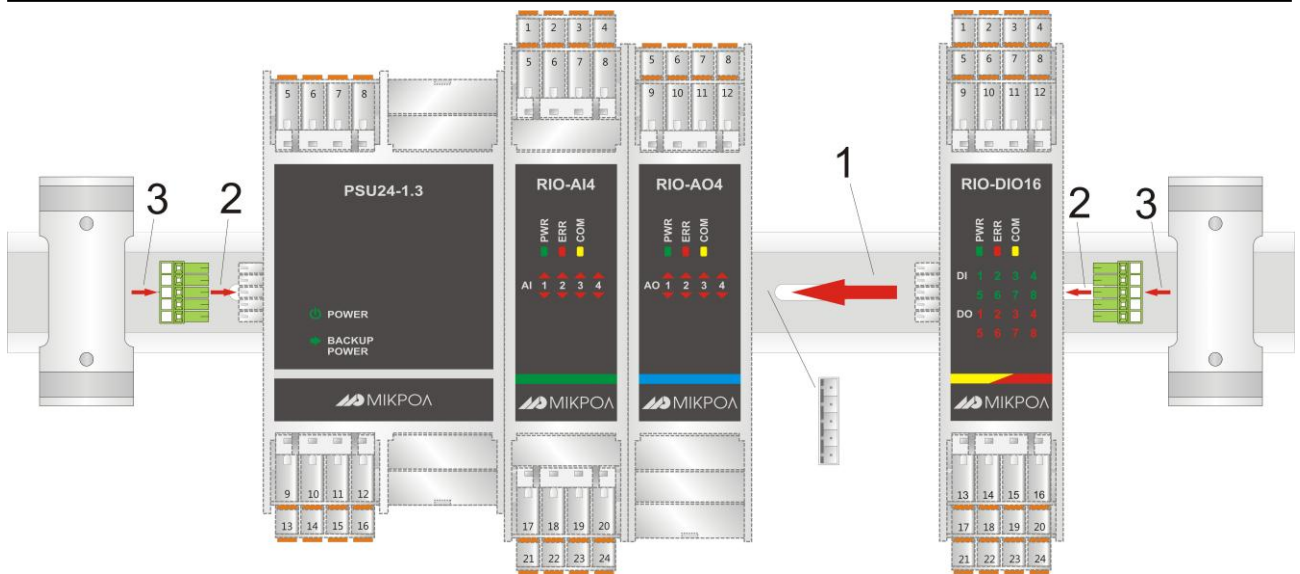
Рисунок 4.2 – Схема соединения блока питания с модулями УСО
