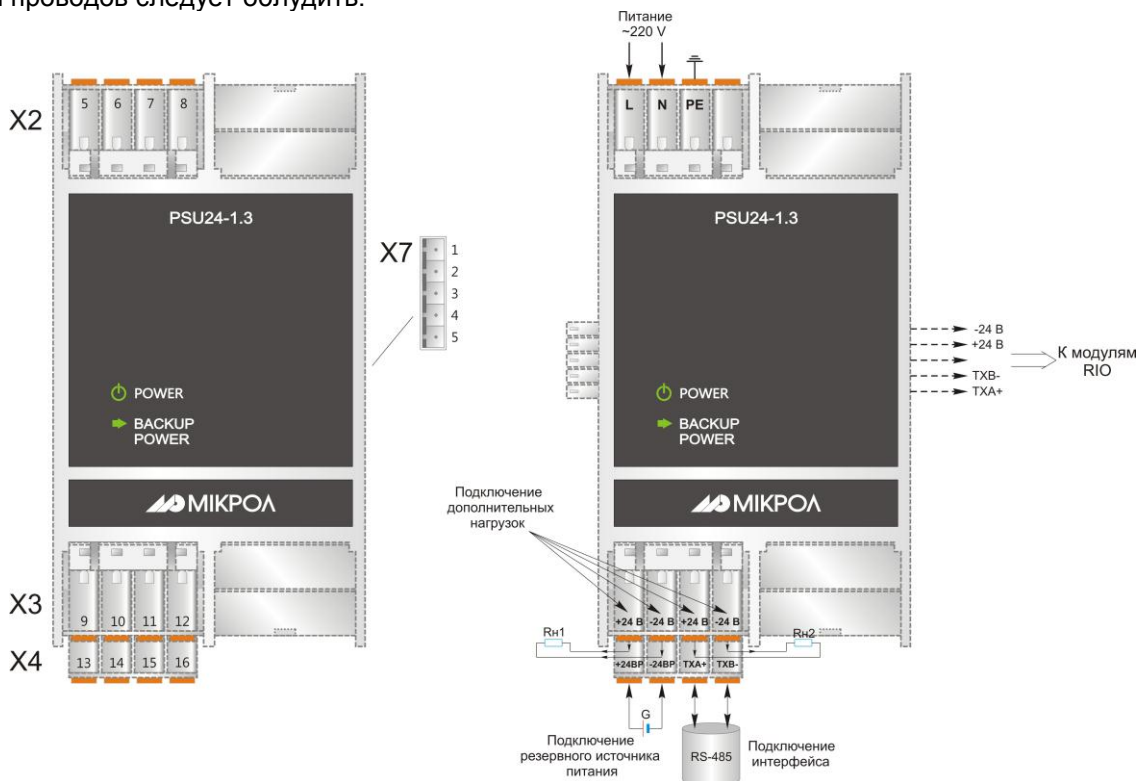
Рисунок 4.3 – Схема внешних соединений PSU24-1.3
