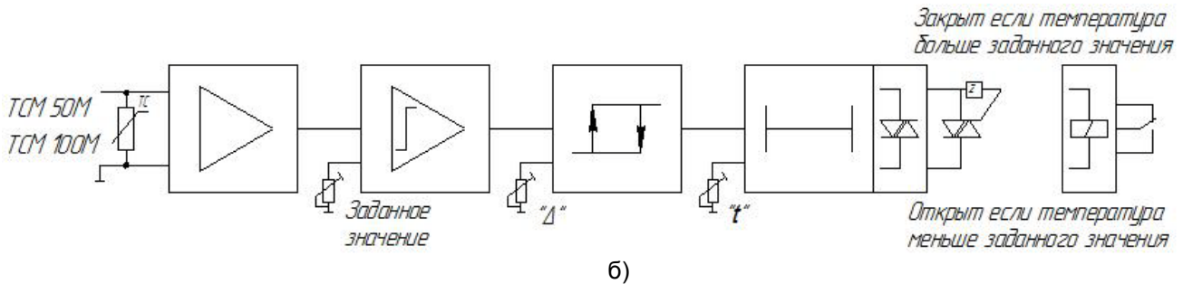
Рисунок 2 – Функциональная схема МИК-1-200
