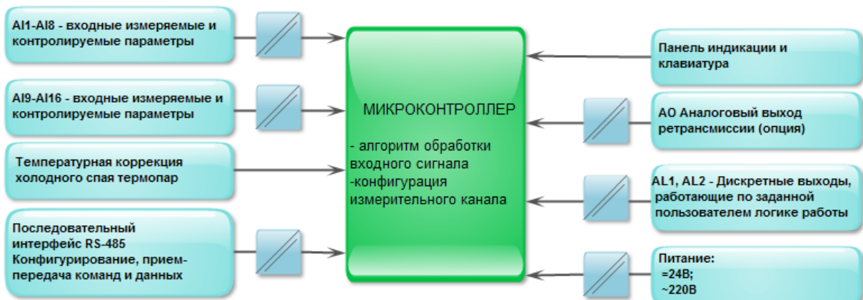
Рисунок 3.2 - Структурная схема индикатора ИТМ-16Н
