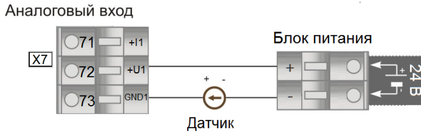
Рисунок Б.2.1 - Подключение к индикатору ИТМ-16Н токовых аналоговых датчиков с пассивными выходами
