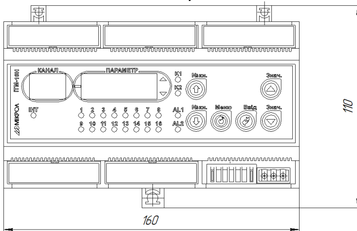
Рисунок А.2 - Габаритные размеры
