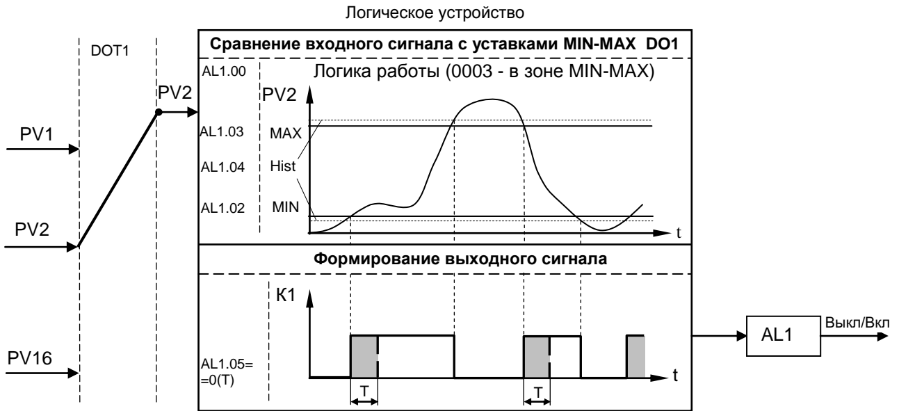
Рисунок 3.7 – Диаграмма работы логических устройств
