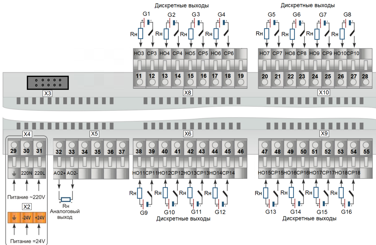
Рисунок Б.4.3 - Схема подключение сигналов модуля расширения MP-51H-15, внешний вид
