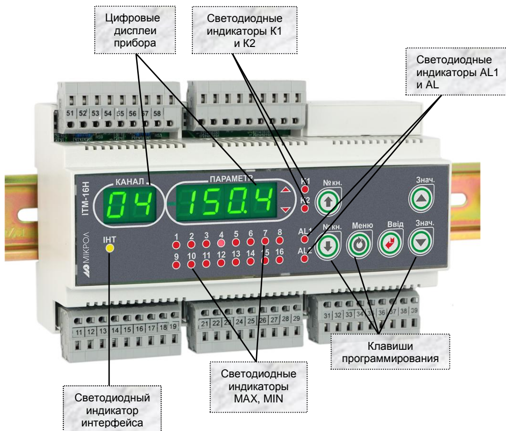
Рисунок 3.1 - Внешний вид передней панели индикатора ИТМ-16Н.
