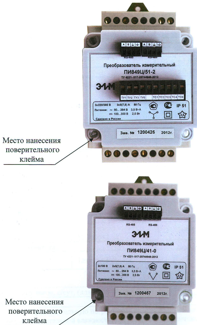
Рисунок 2 – Внешний вид ПИ849Ц
