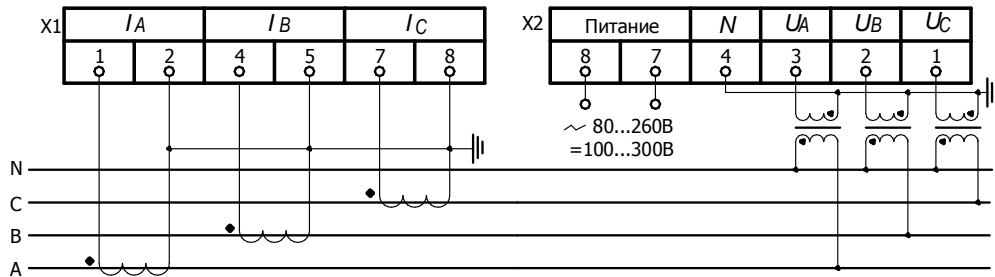
Рисунок В.13 - Схема подключения ПИ849Ц/1Х-Х, ПИ849Ц/3Х-Х, ПИ849Ц/5Х-Х к четырехпроводной сети
