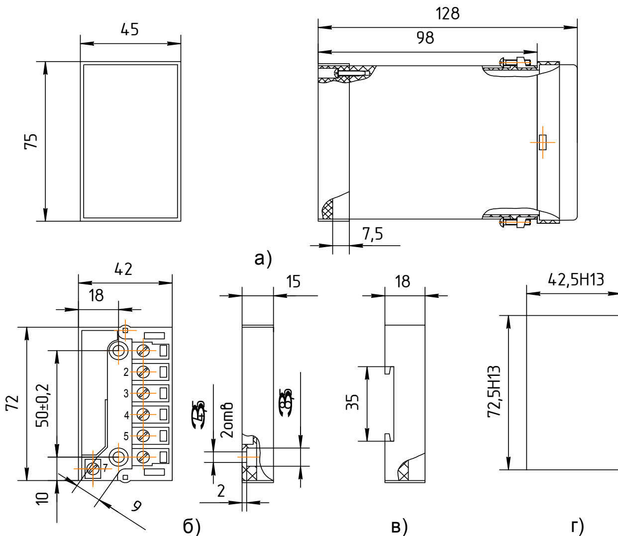
а) общий вид реле; б) колодка для установки реле утопленным монтажом, выступающим монтажом на плоскость и подсоединения проводов под винт; в) колодка для установки реле на рейку DIN 35 мм; г) разметка панели для установки реле утопленным монтажом
