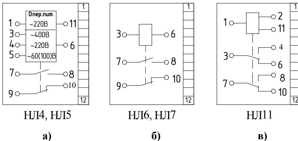
Рисунок 3 – Схемы подключения реле
